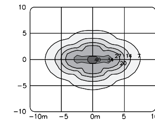
Isolux L.P.H. = 4m
