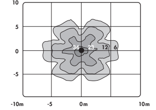
Isolux L.P.H. = 4m
